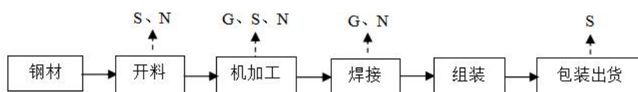
图 3-3 印刷包装机械生产工艺及产污环节流程图 (S 为固体废物；N 为噪声；G 为废气)
